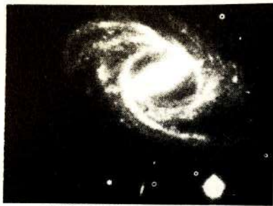
NGC 2523
